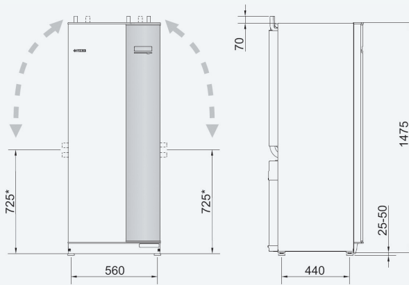
NIBE F1155
