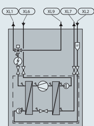
NIBE F1155
